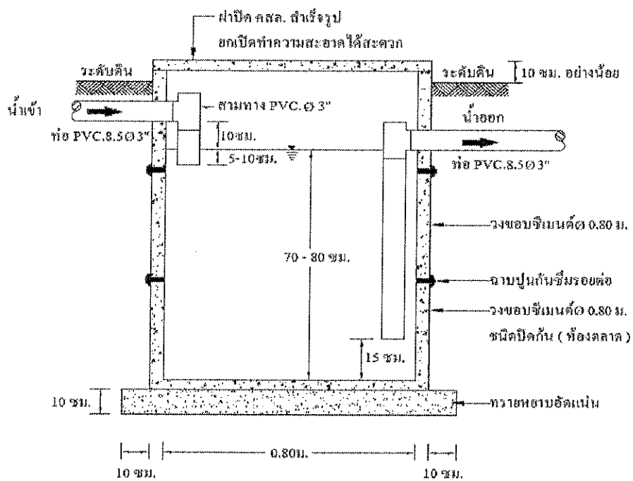
แปลนภาพตัดขวางบ่อดักไขมันแบบวงขอบซีเมนต์
