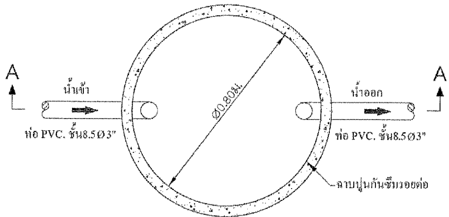
แปลนภาพด้านบนของบ่อดักไขมันแบบวงขอบซีเมนต์
